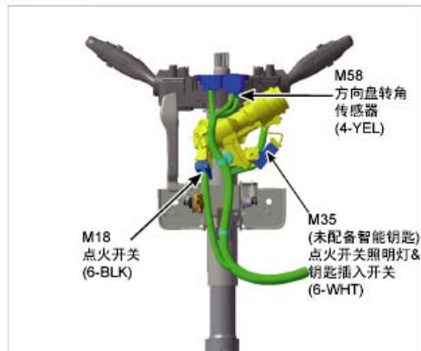
61.转向柱
